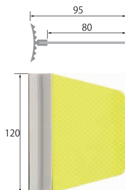
FD-120
