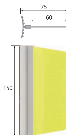
FD-150
