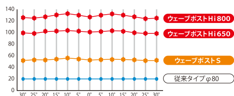
● 1基当たりの総反射輝度値データ
