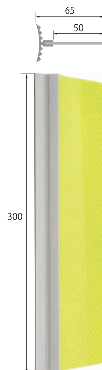
FD-300
