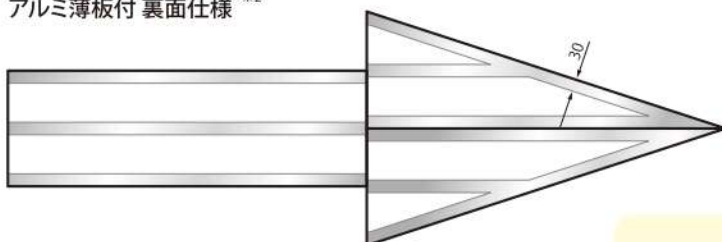
裏面 プチル系粘着テープ用アルミ薄板配置図
