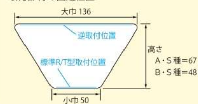
取付部材の固定位置
