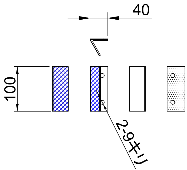
製品図 1:4
